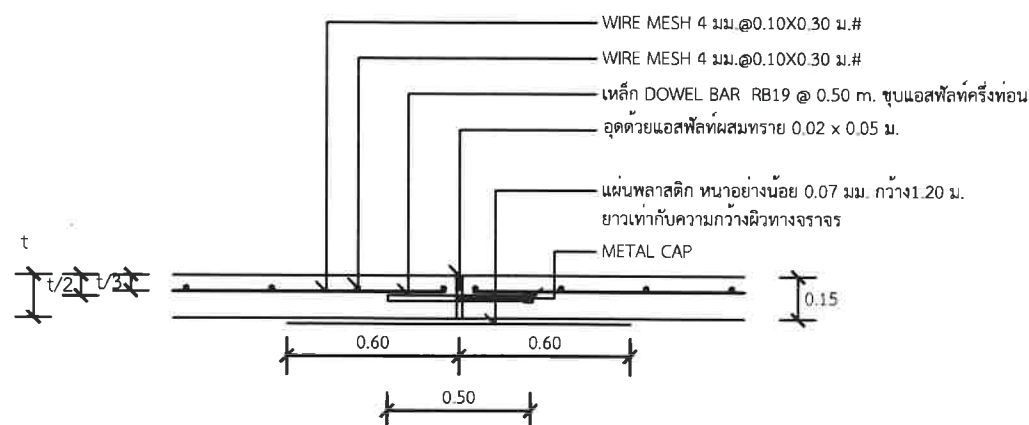
แบบขยาย ก EXPANSION JOINT ทุกระยะไม่เกิน 50 เมตร NOT TO SCALE
