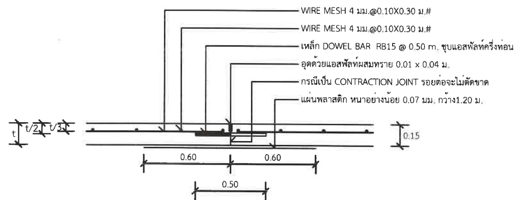
แบบขยาย ข CONSTRUCTION JOINT และ CONTRACTION JOINT ทุกระยะ 10 เมตร NOT TO SCALE
