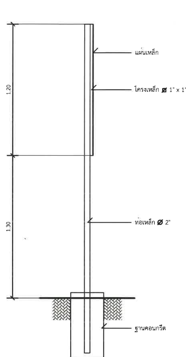
รูปดานขาง
