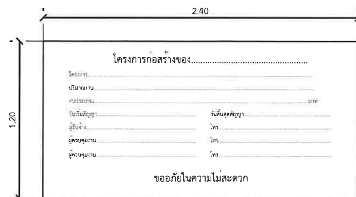
แบบขยายข้อความป้ายไวนิล
