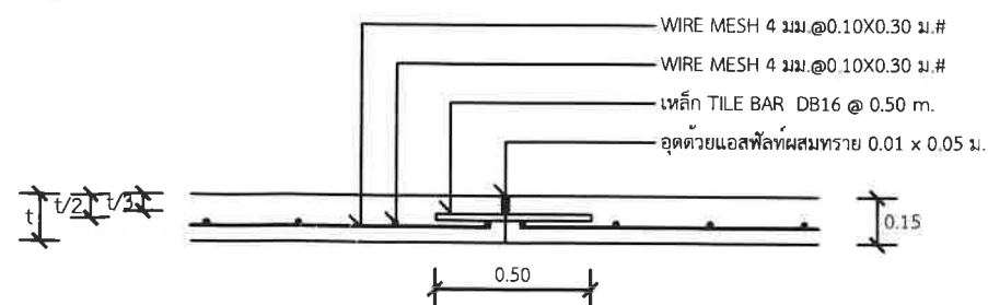
แบบขยาย ค LONGITUDINAL JOINT NOT TO SCALE
