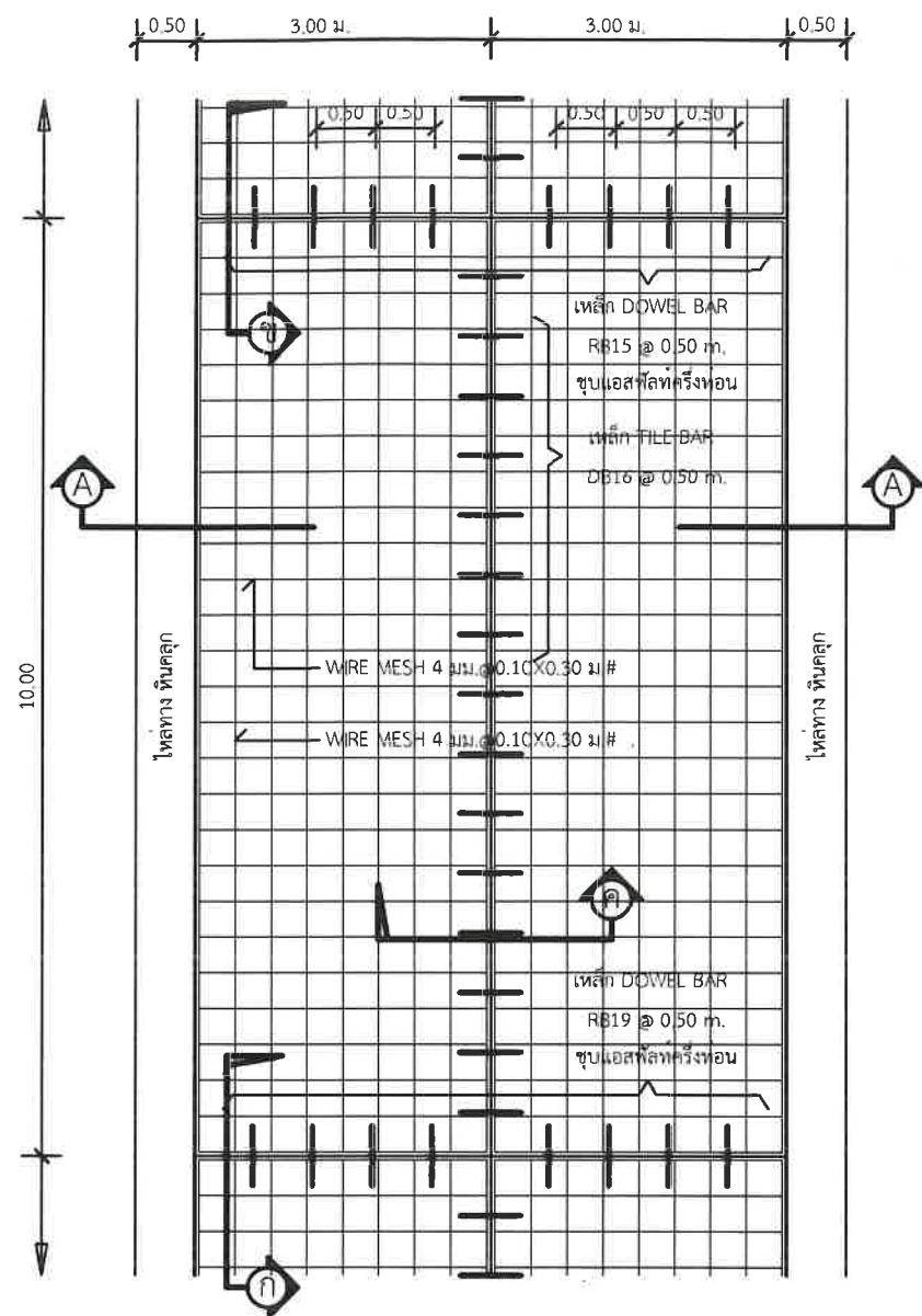
แปลนพื้นถนน NOT TO SCALE
