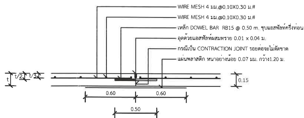
แบบขยาย ข CONSTRUCTION JOINT และ CONTRACTION JOINT ทุกระยะ 10 เมตร
