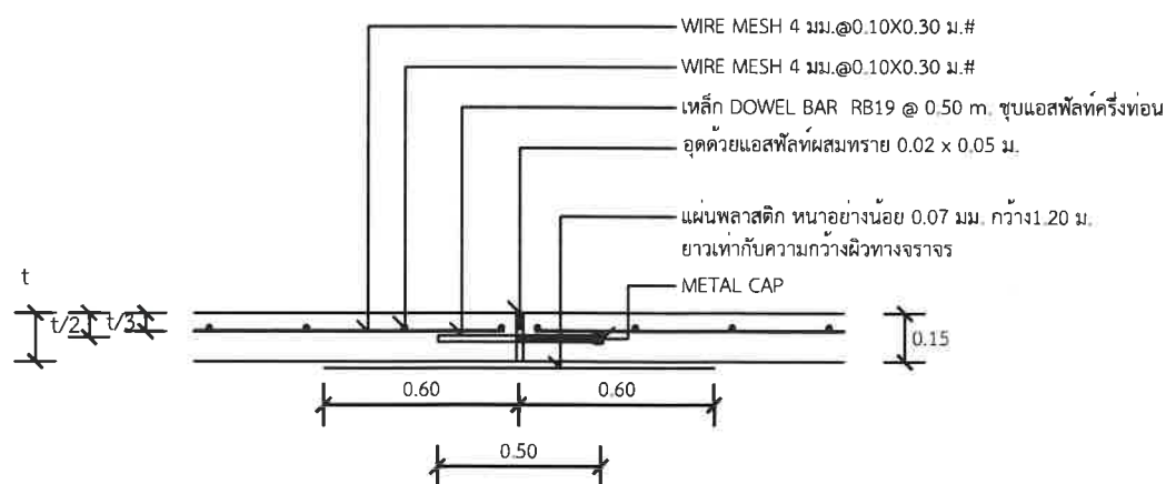
แบบขยาย ก EXPANSION JOINT ทุกระยะไม่เกิน 50 เมตร
