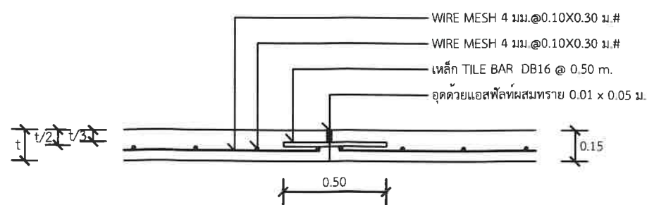
แบบขยาย ค LONGITUDINAL JOINT
